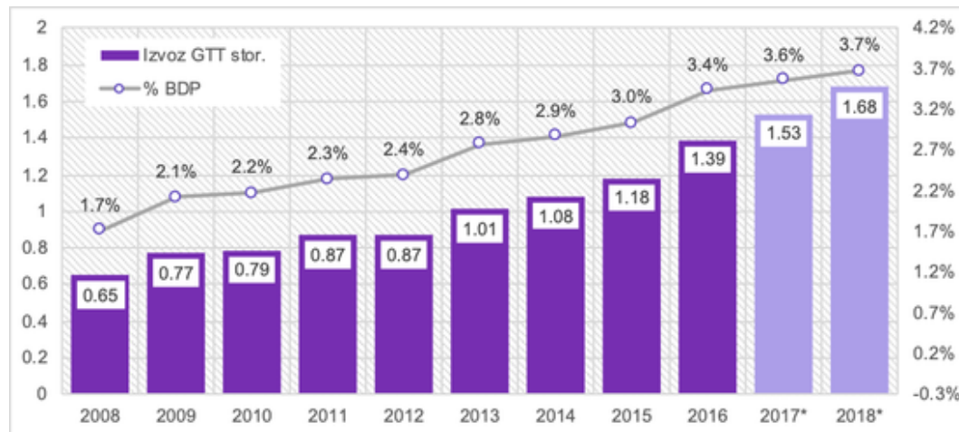
Slika 1: Skupni izvoz nabora GTT storitev iz Slovenije (v mlr EUR) in delež v BDP (%) v obdobju 2008 – 2018
