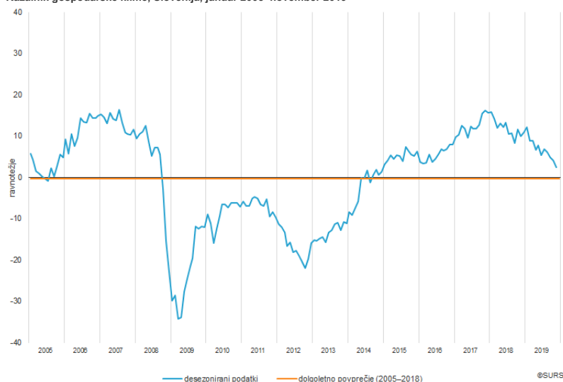
Kazalnik gospodarske klime, Slovenija, januar 2005–november 2019
