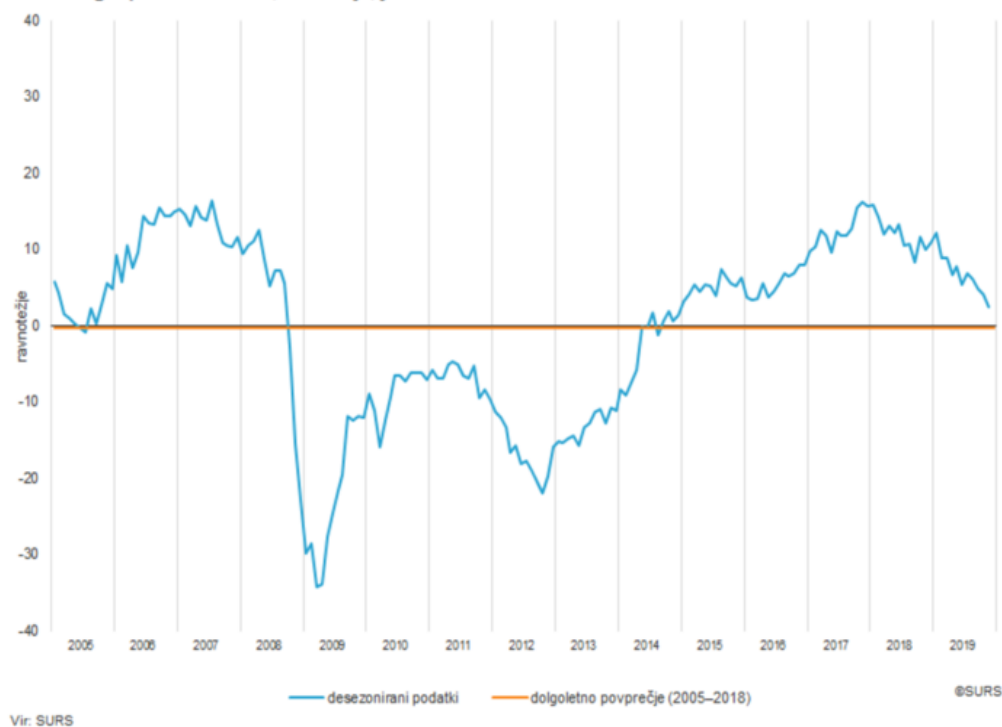
Kazalnik gospodarske klime, Slovenija, januar 2005–november 2019
