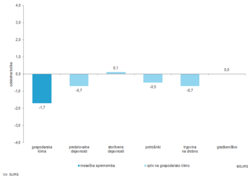
Vpliv posameznih kazalnikov zaupanja na mesečno spremembo gospodarske klime, Slovenija, november 2019
