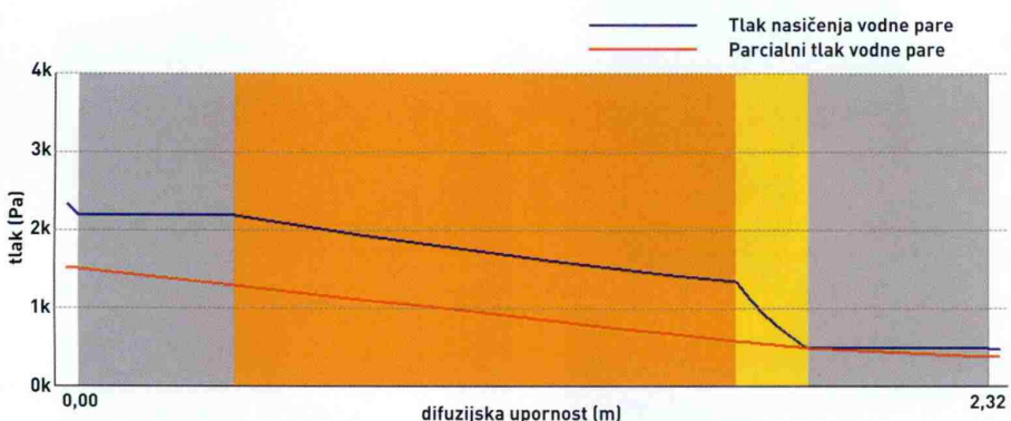
Graf 2: Porobeton + mineralna volna + 'ZSPVDU'
