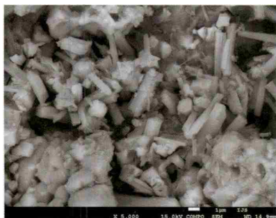
Mikroskopski posnetek hidratacijskih produktov cementa
