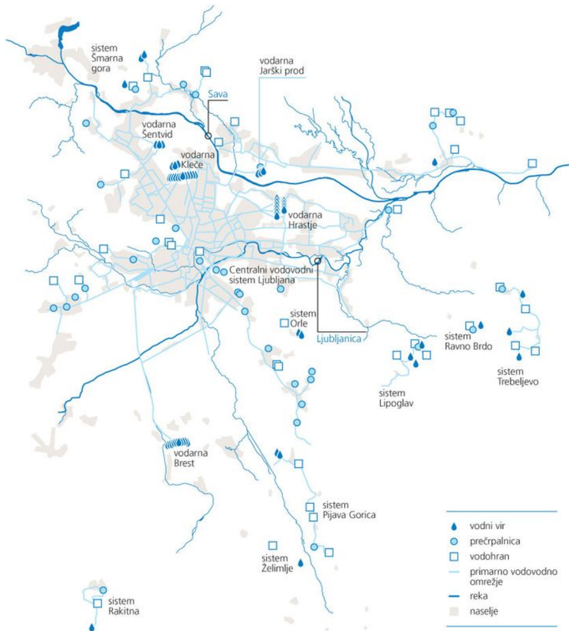
Vodovodni sistemi v Ljubljani in okolici v upravljanju JP VOKA SNAGA. Foto: VOKA Snaga
