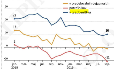
Kazalnik zaupanja
