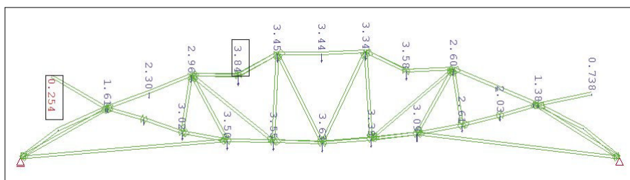
Slika 9 • Izris navpičnih upogibkov (mm) s programom Sofistik
