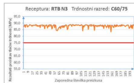
Slika 29: Rezultati preizkusov tlačnih trdnosti betona C60/75, XC4, XD3, Dmax 32, S4, PV-II.
