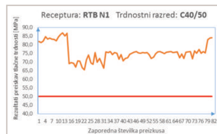
Slika 27: Rezultati preizkusov tlačnih trdnosti betona C40/50, Dmax 32, XC4, XD3, S4, PV-II.
